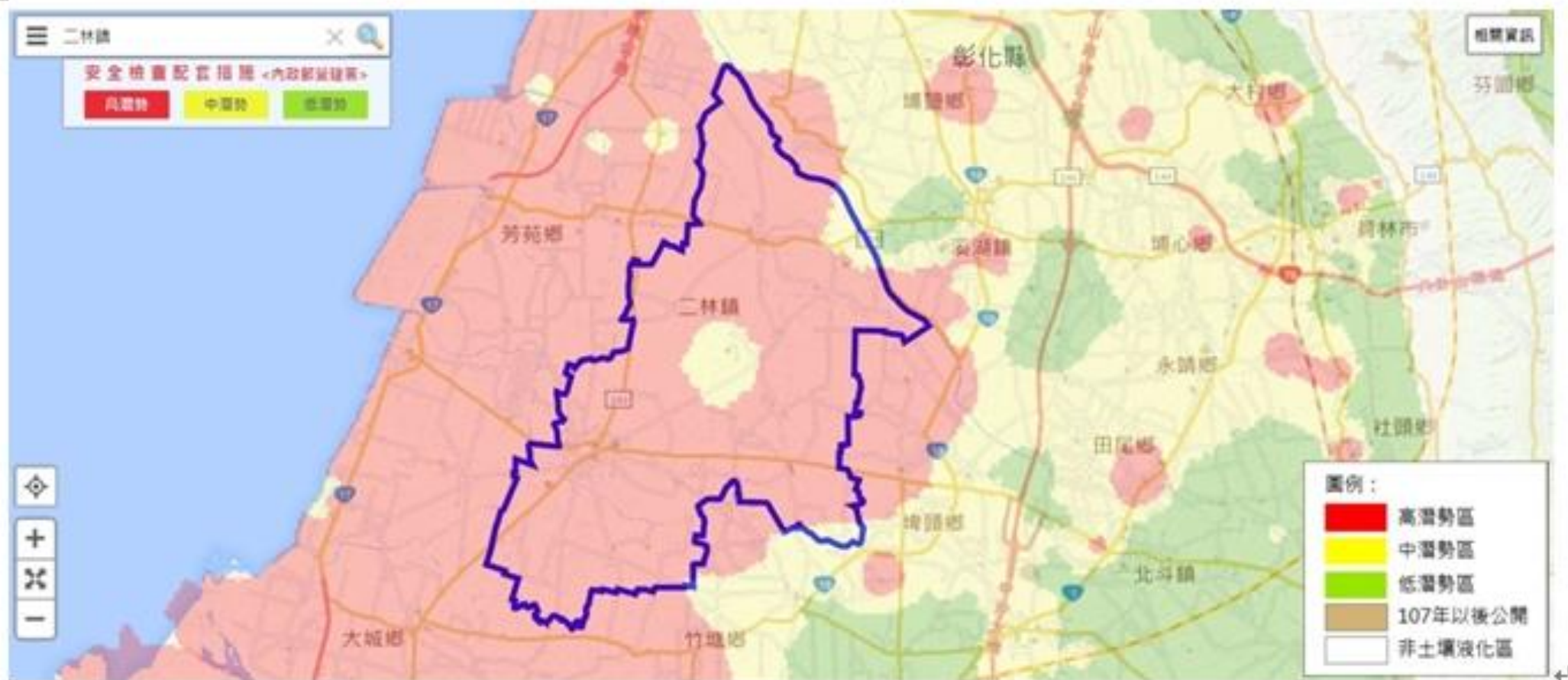
二林鎮土壤液化潛勢區分布圖
