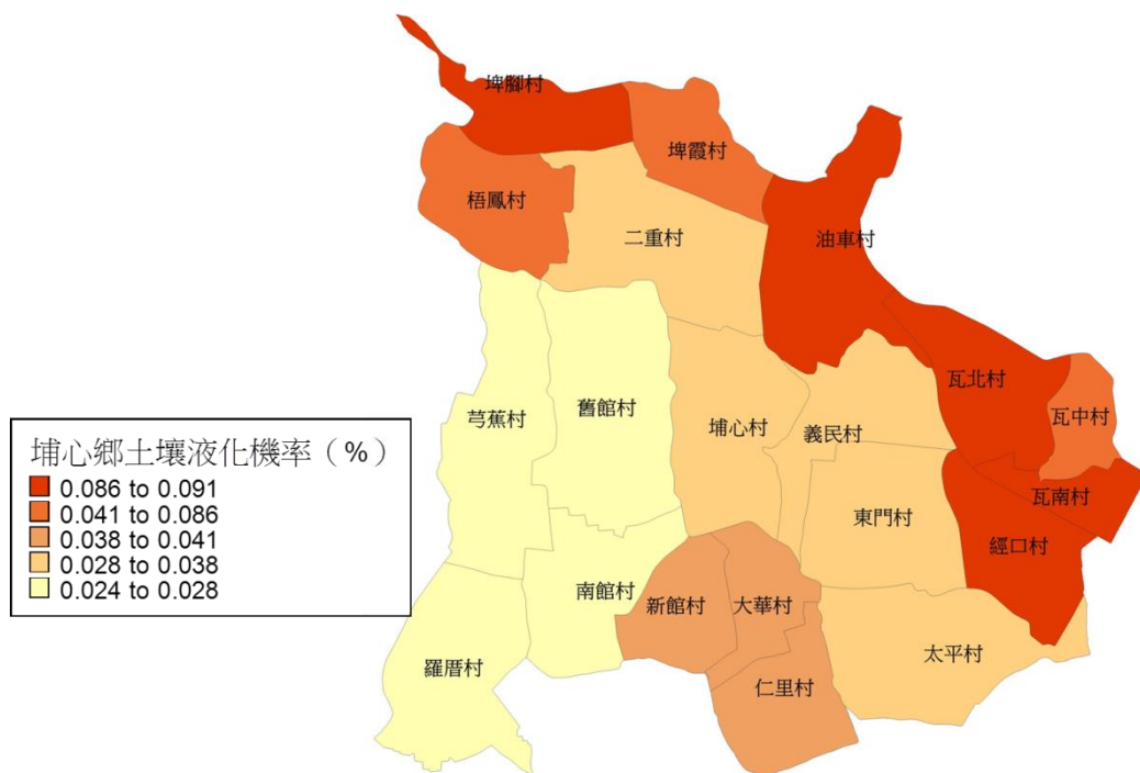
圖 1-3-10 土壤液化分布圖
