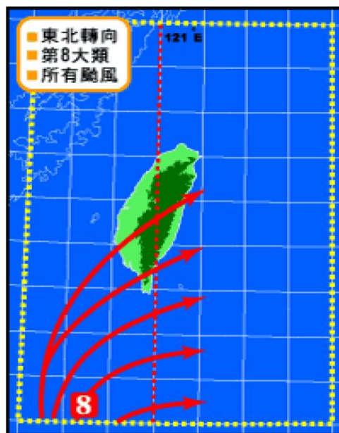
圖 1-3-5 第 8 類颱風路徑
