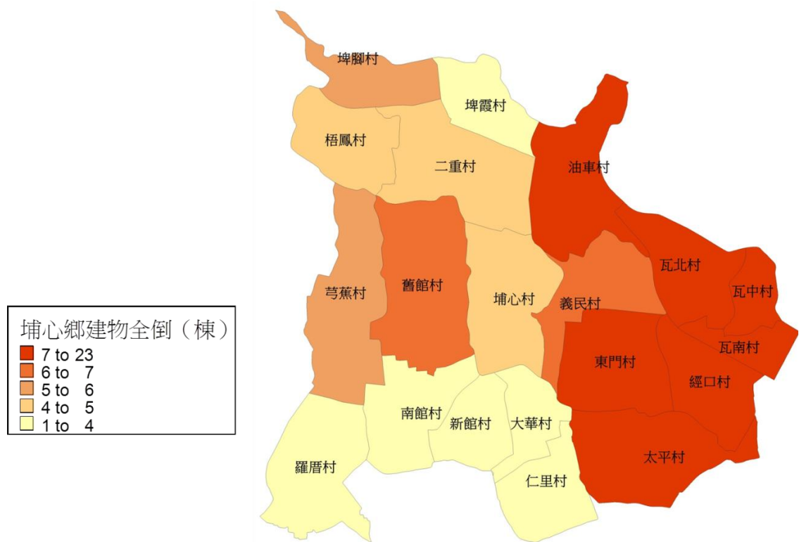
圖3-12 建物全倒分布圖
