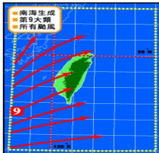
圖 3-6 第 9 類颱風路徑
