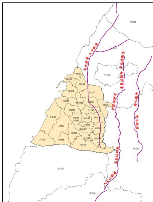
圖3-8 彰化縣附近斷層分布圖
