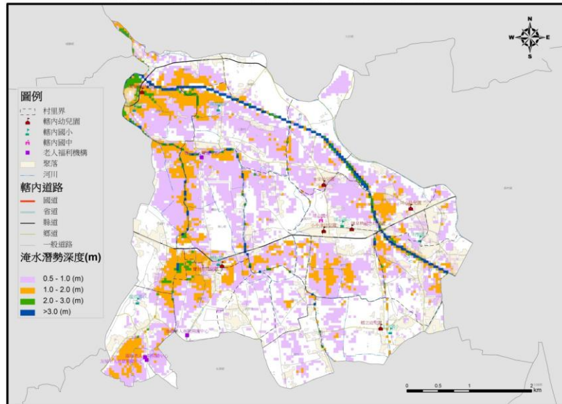
彰化縣埔心鄉水災災害潛勢圖 (350mm/24hr)
