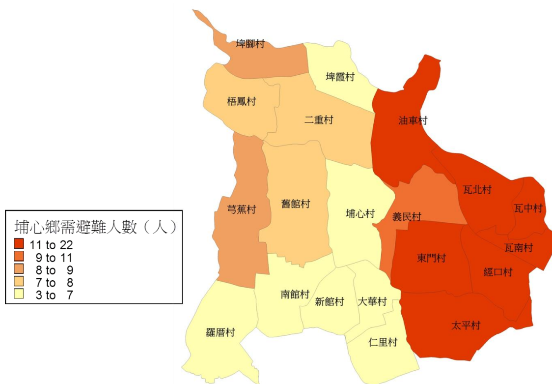
圖3-9 需避難人數分布圖
