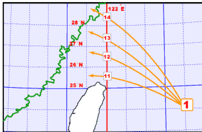
圖 3-1 第 1 類颱風路徑
