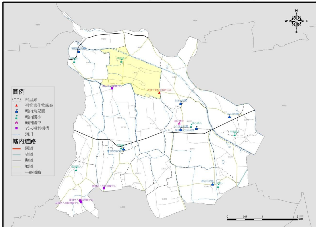
圖 3-13 埔心鄉毒化災害潛勢圖
