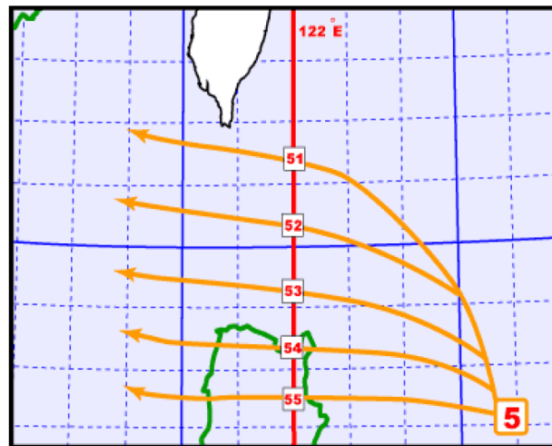
圖 3-3 第 5 類颱風路徑
