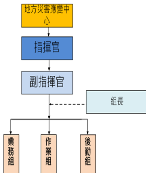
圖2-3 災害應變中心組織架構
