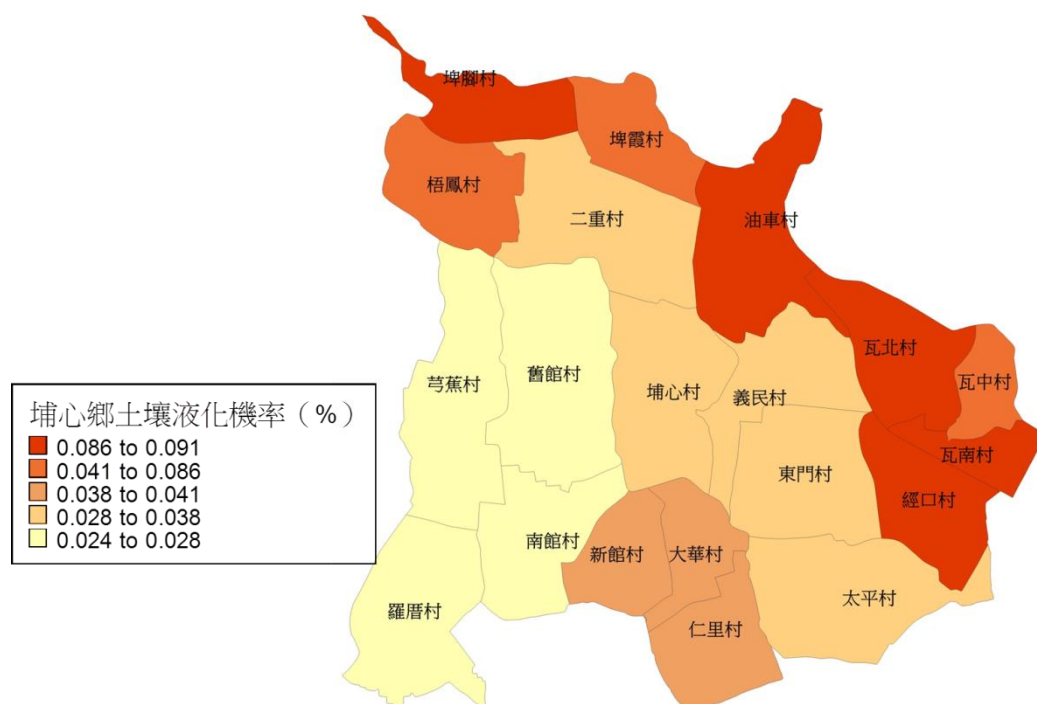
圖3-10 土壤液化分布圖
