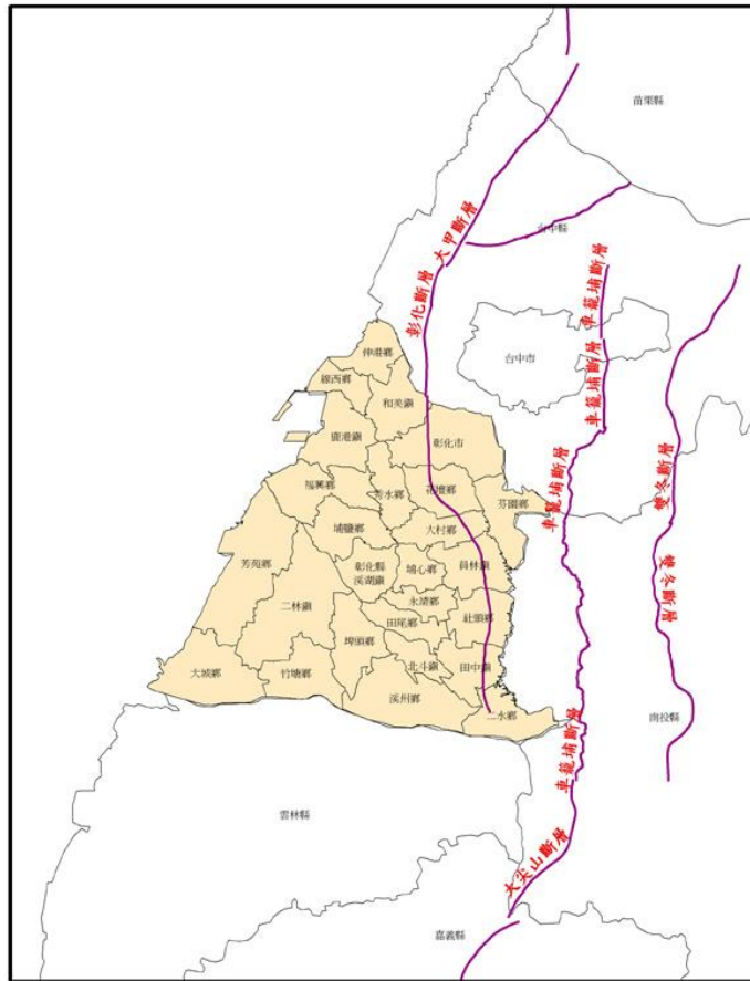
圖3-8 彰化縣附近斷層分布圖
