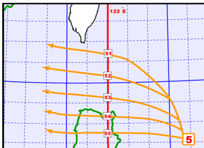
圖 3-3 第 5 類颱風路徑
