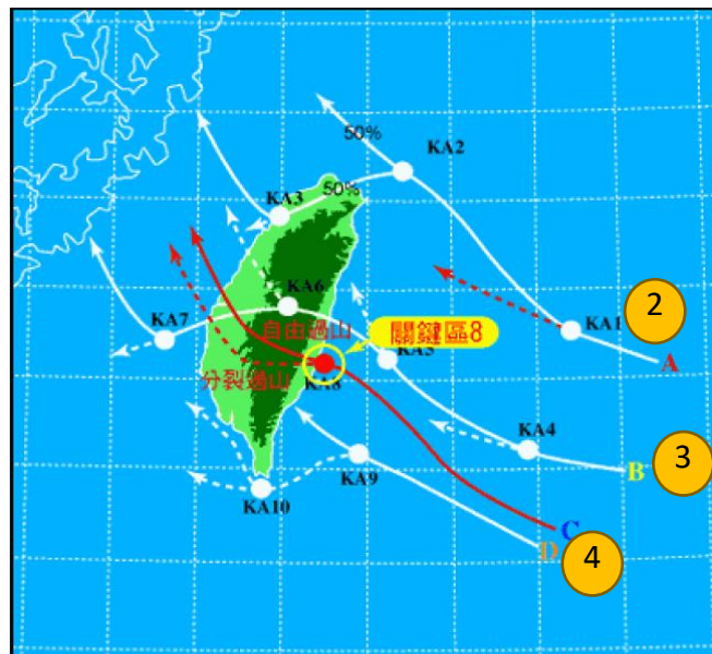
圖 3-2 第 2、3、4 類颱風路徑
