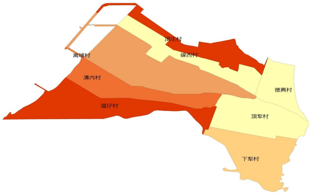
圖3-10 土壤液化分布圖
