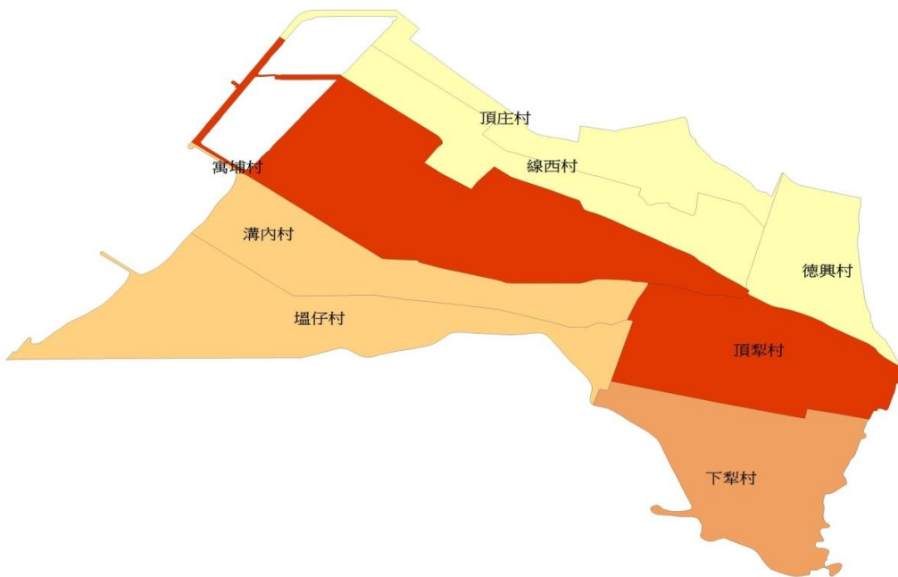
圖3-11 建物半倒分布圖
