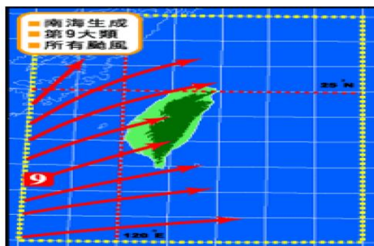
圖 3-6 第 9 類颱風路徑
