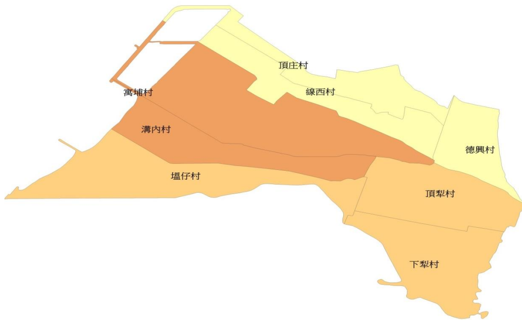
圖3-12 建物全倒分布圖
