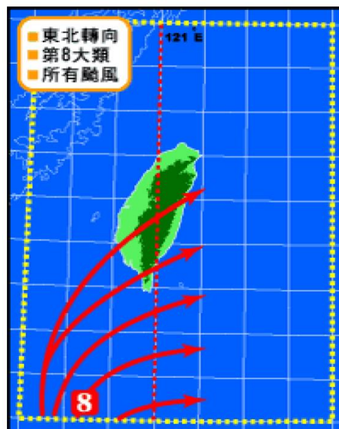
圖 3-5 第 8 類颱風路徑
