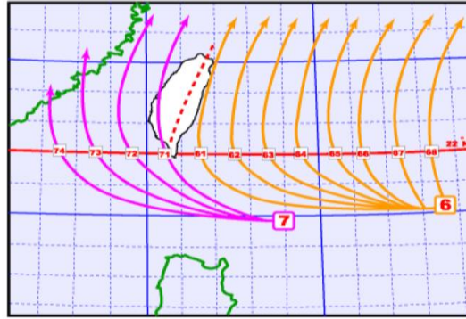
圖 3-4 第 6、7 類颱風路徑
