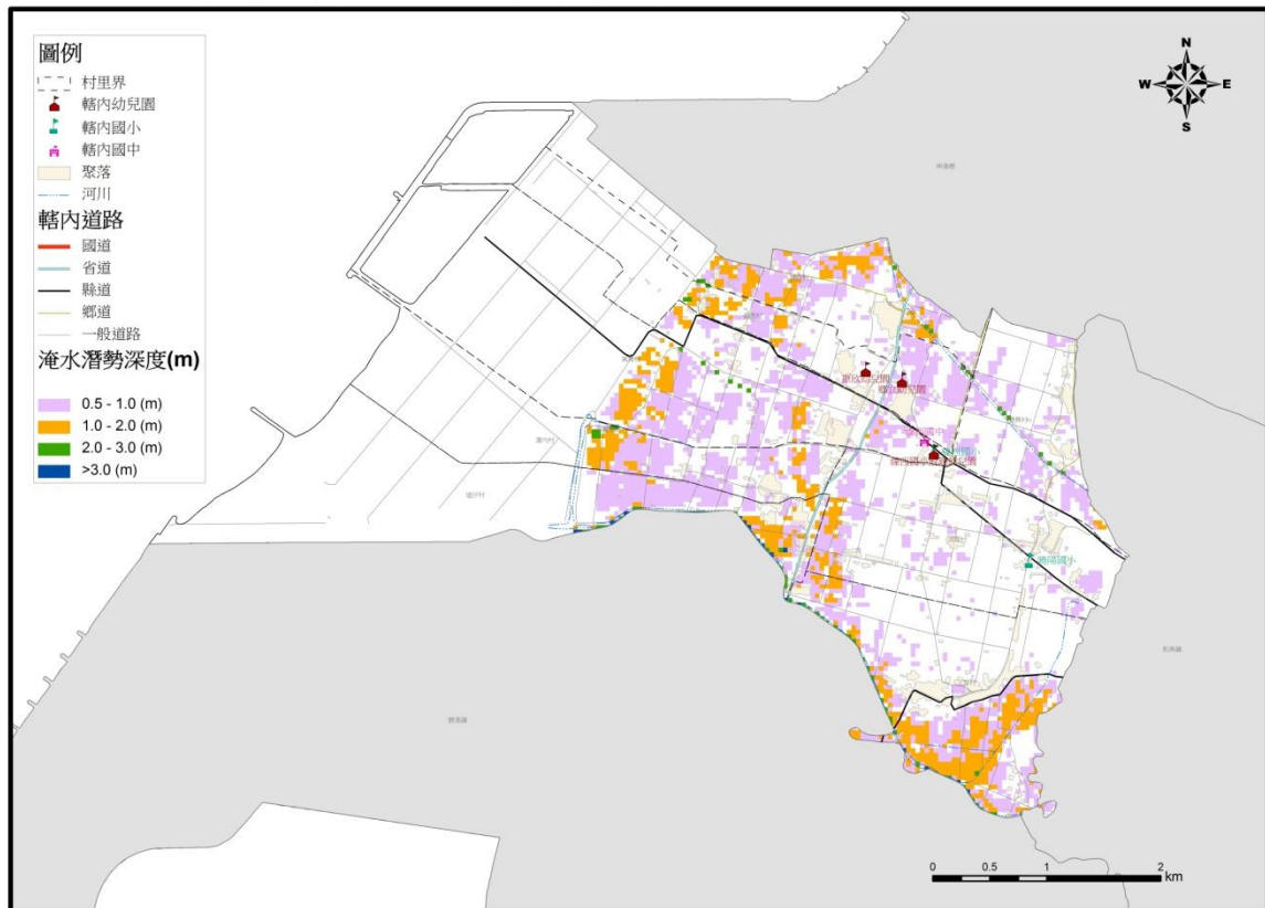
圖3-7 線西鄉淹水潛勢圖
